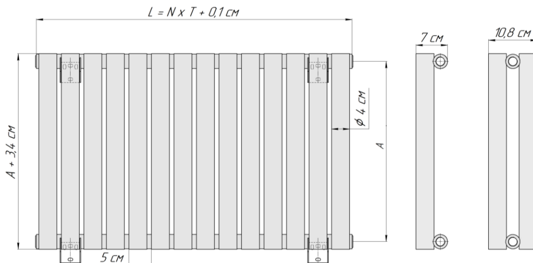
Рис. 1. «Гармония А40», где: А – межцентровый размер, см; Т – шаг (Т = 5 см); N – количество секций; L – габаритная длина, см.
